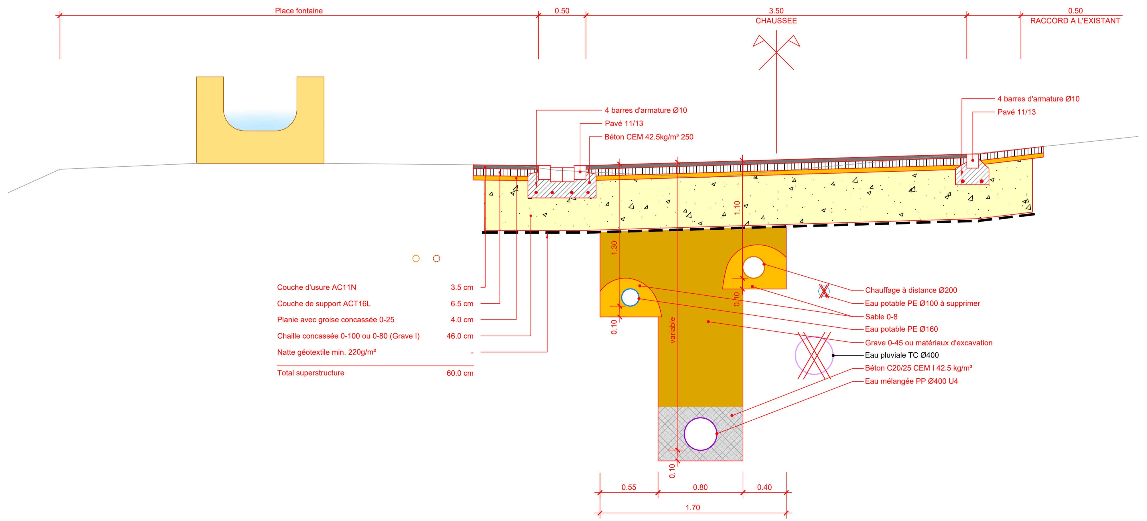
Coupe type 3 1:20
