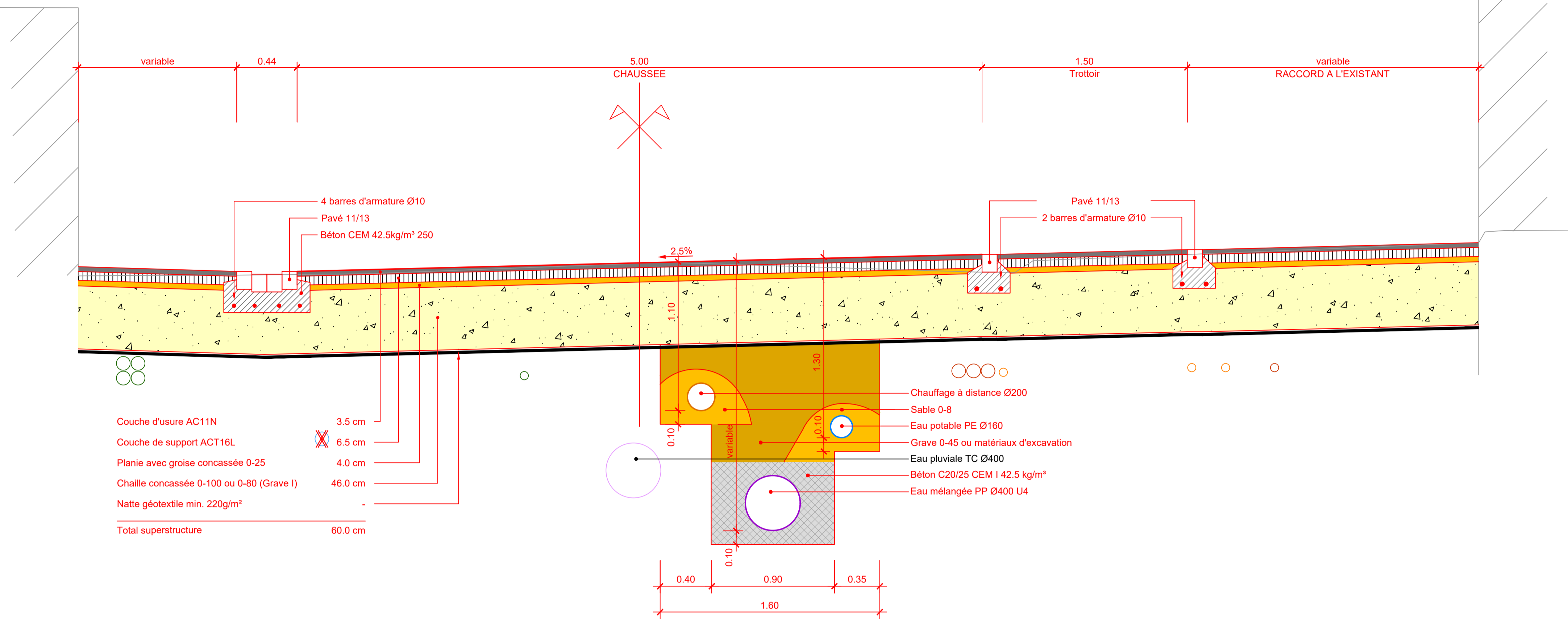
Coupe type 3 1:20
