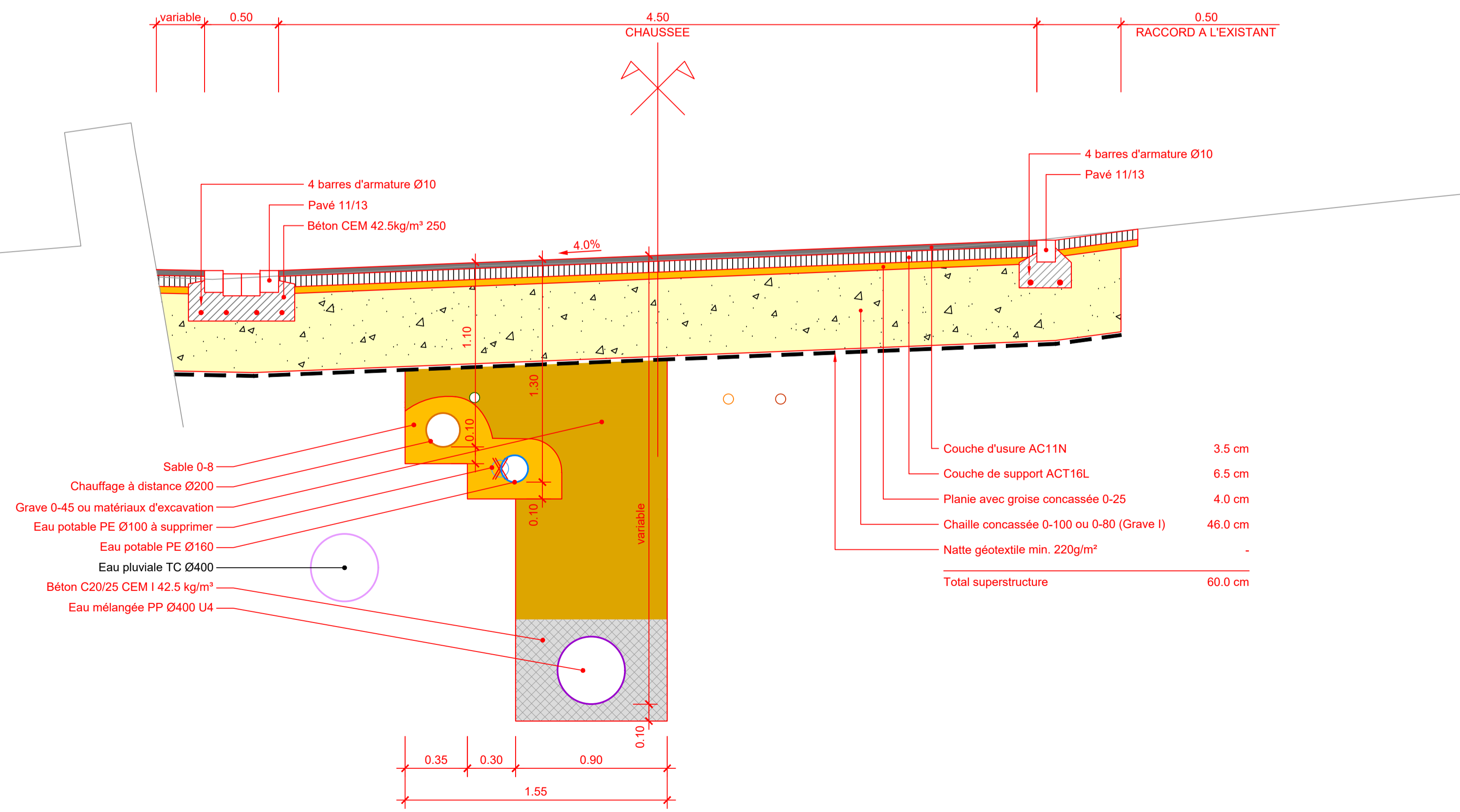
Coupe type 2 1:20
